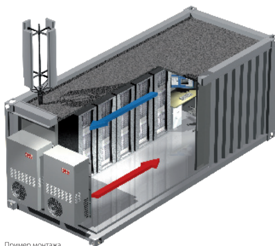
Пример монтажа
