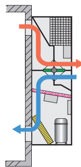
Естественное охлаждение
