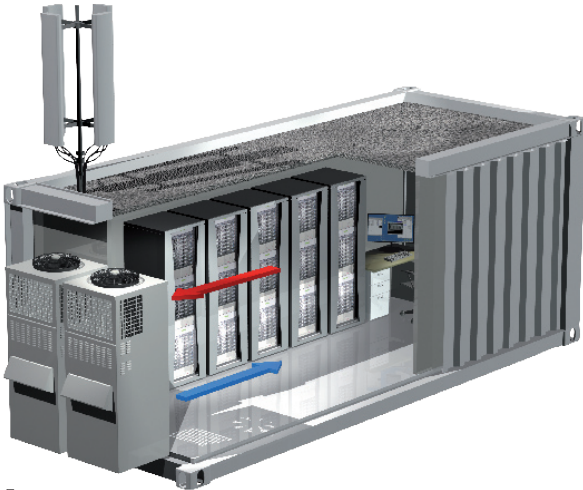
Пример монтажа
